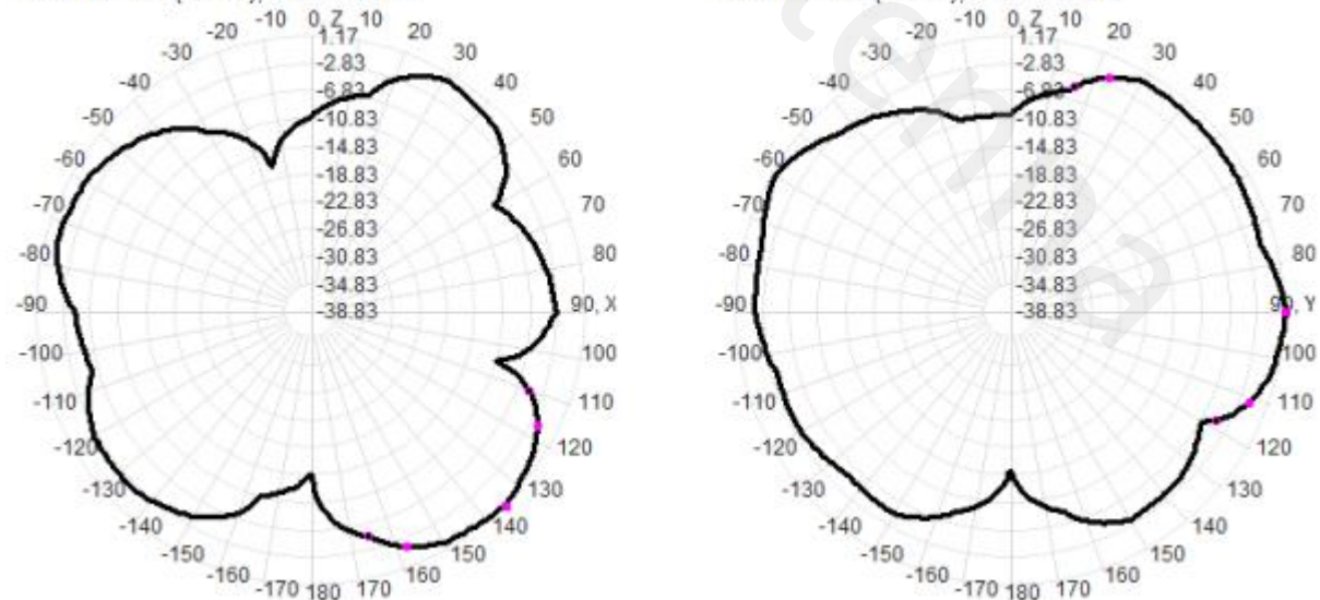
780.0MHz Total(E1-XZ), Max= 0.98dBi
